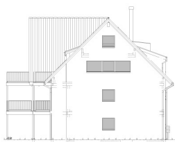
Ostfassade
