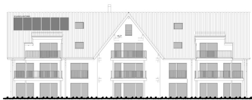
Südfassade
